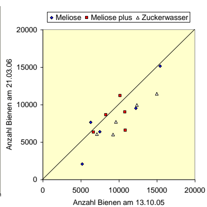
Abb. 3: Die Überwinterung der Jungvölker in 2005/2006 am Standort Wald (320 m N.N.). Das Futtermittel hat keinen Einfluss.
