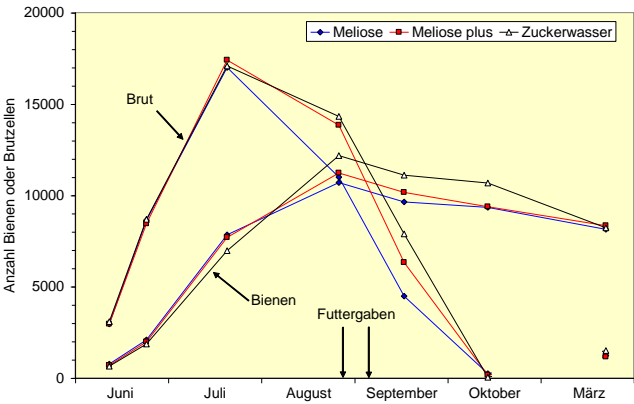
Abb. 2: Die Entwicklung von Jungvölkern in 2005/2006 am Standort Wald (320 m N.N.). Mittelwerte von je 5 Völkern.
