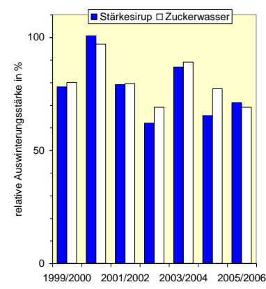
Abb. 4: Die relative Auswinterungsstärke der mit Sirup und Zuckerwasser gefütterten Völker in 1999/2000 bis 2005/2006. Mittelwerte von allen an 3-10 Standorten aufgestellten Völkern.
